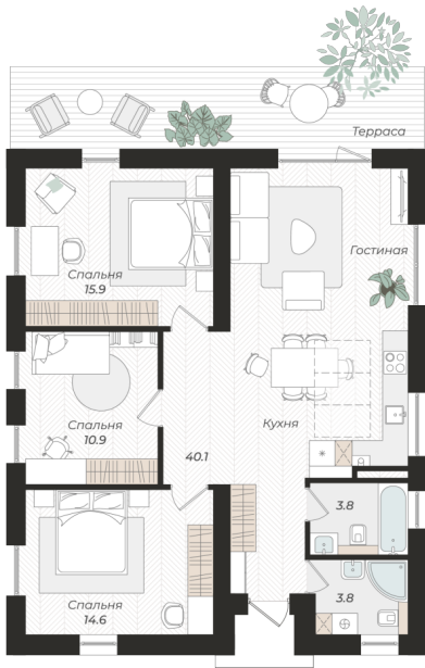
Планировка
